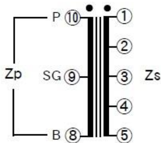
端子接続図
