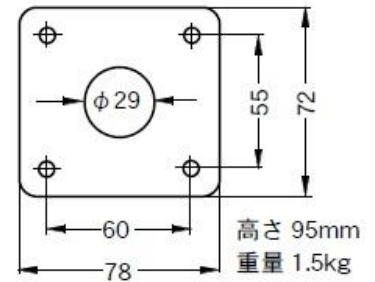
外形図
