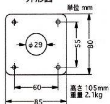
外形図
