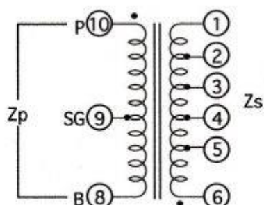
端子接続図
